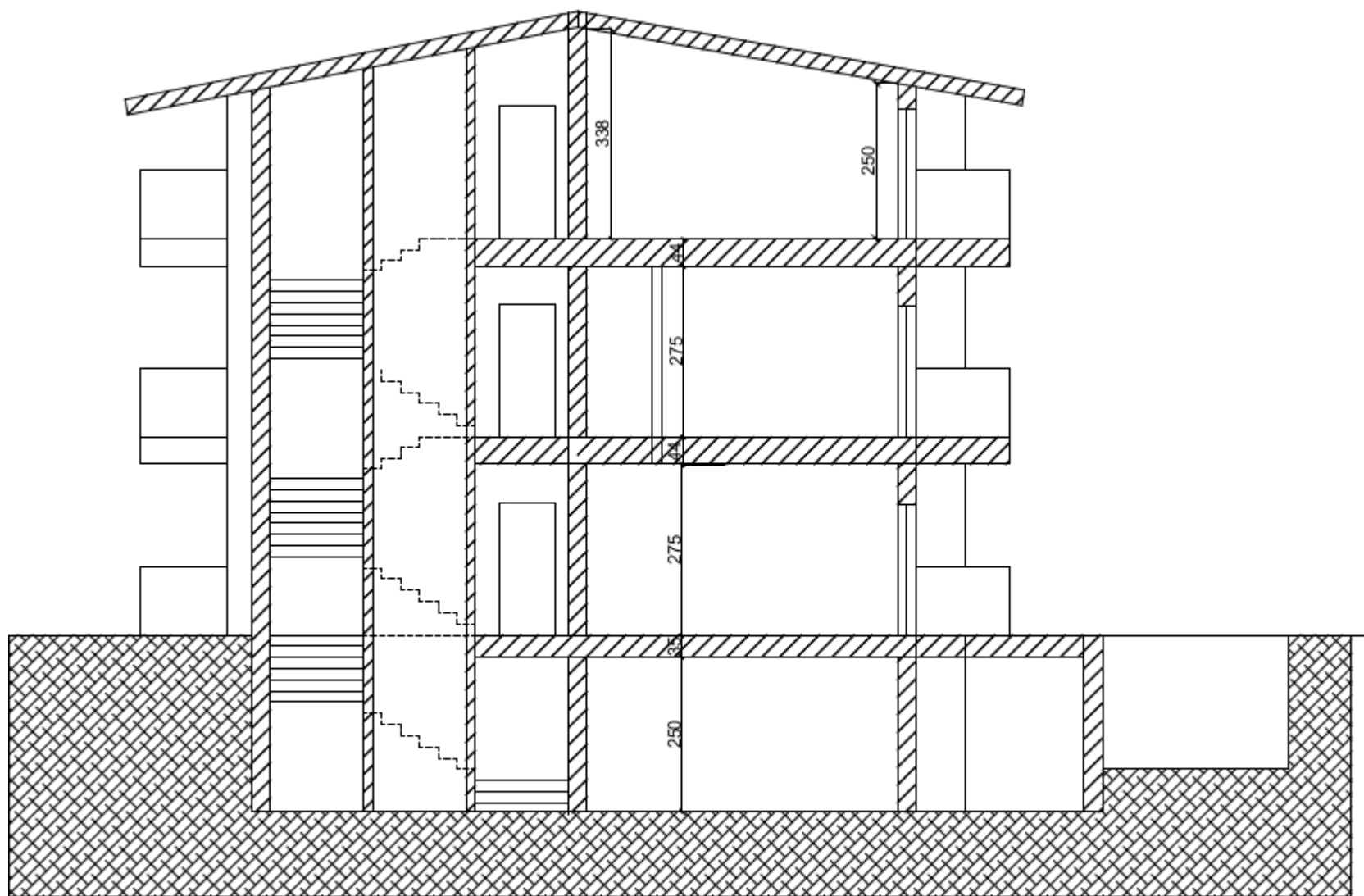
Sezione Trasversale
